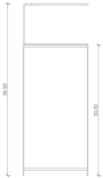
CONTENITORE + PORTAROTOLO
