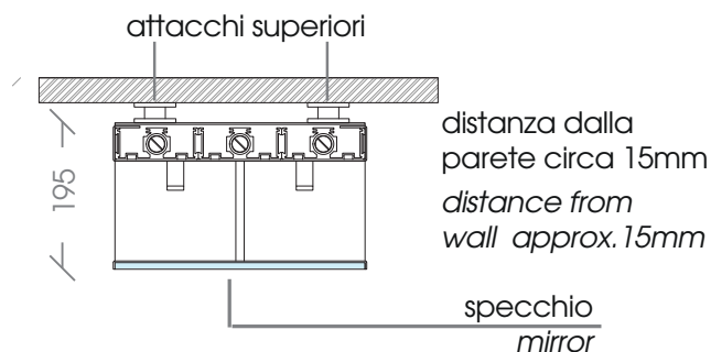
sezione
